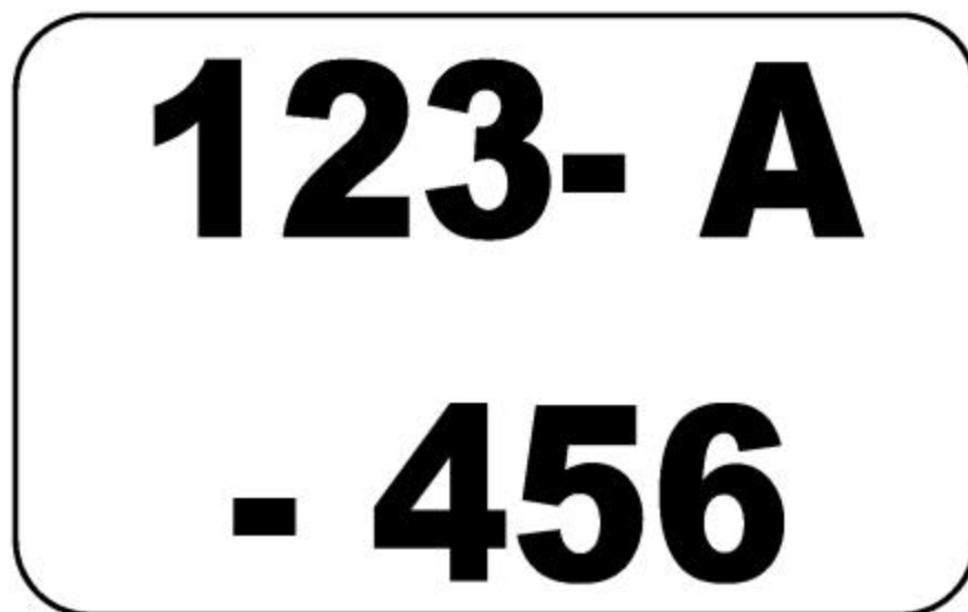
Izgled tablice, dimenzije 240 mm x 130 mm x 1 mm
